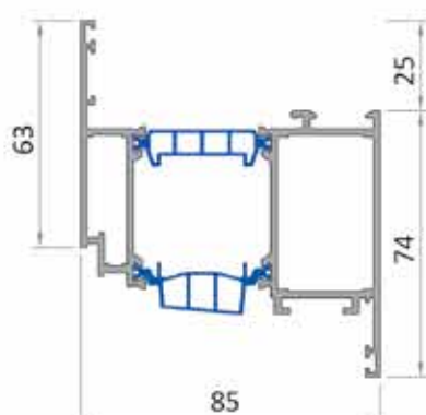
Door sash profile RP 85.25 2210 g/m
