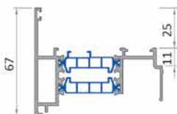
Door sash profile RP 85.27 2270 g/m
