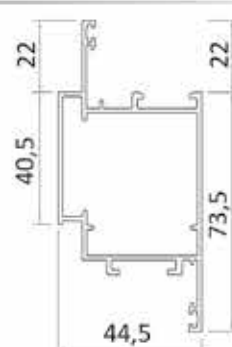
Крыло врата RP 2008 1030 гр/м
