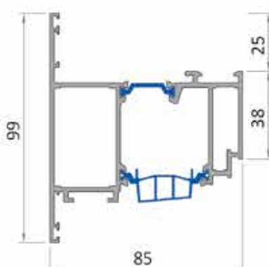
Door sash profile RP 85.27 2270 g/m
